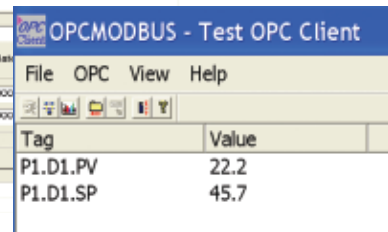
OPC client
