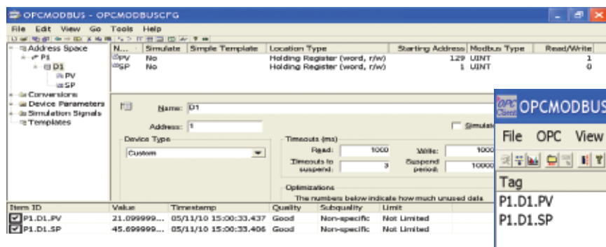
OPC server
